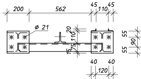
Ansicht Stirnseite
